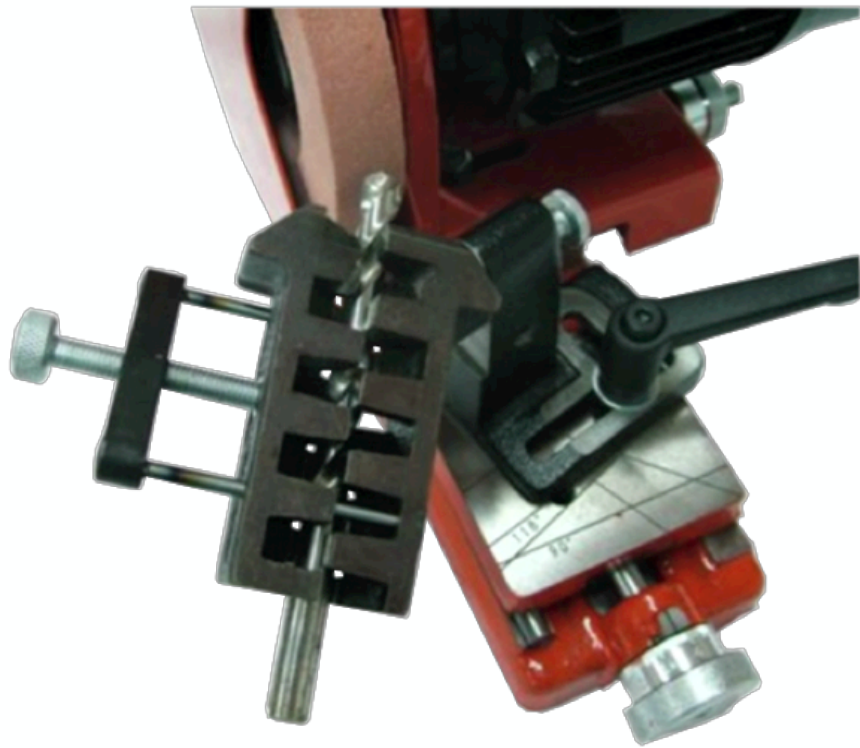
Vista del portabrocas
