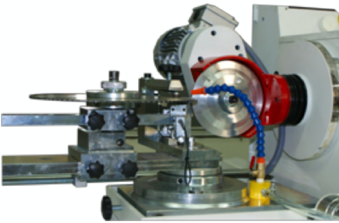
Afilado de la cara
