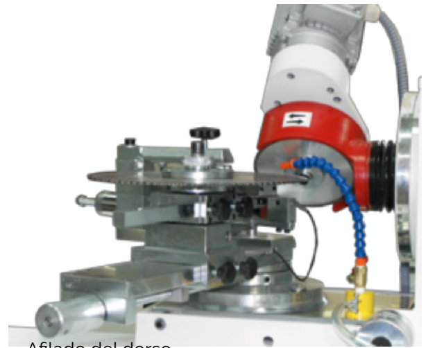
Afilado del dorso
